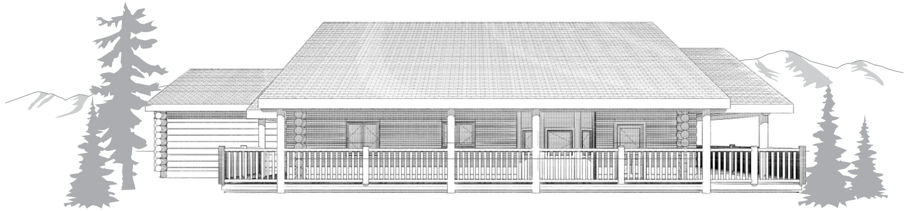
RIGHT ELEVATION
